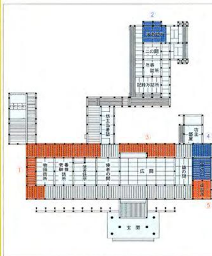
現存する本丸御殿平面図
