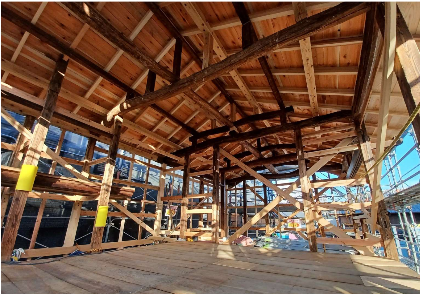
旧栄養食配給所住宅棟の施工状況
