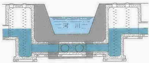
河川の下を横断する下水管
