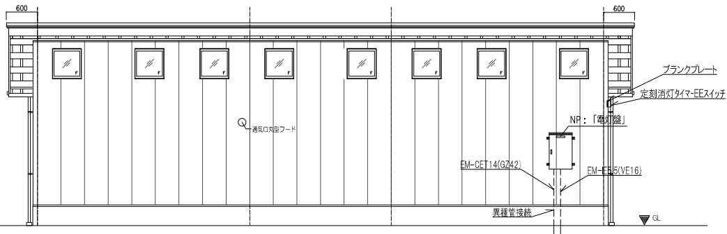
南立面図
