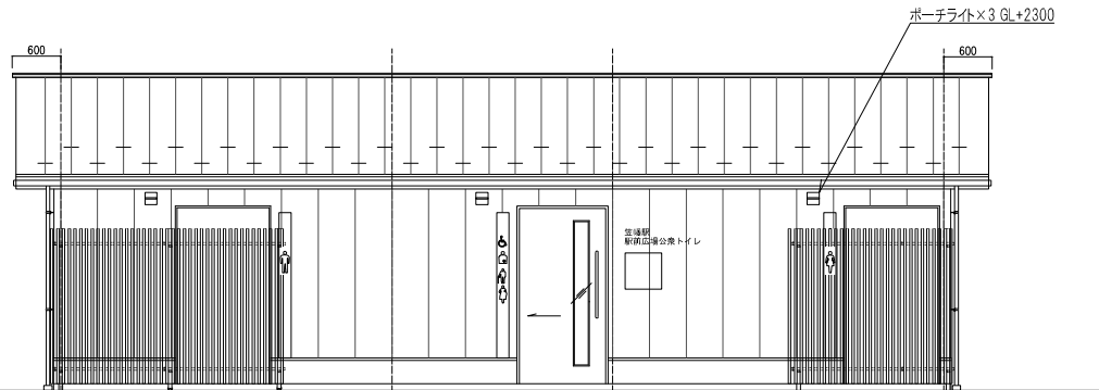
南立面図
