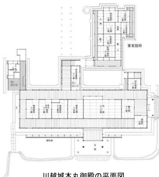
川越城本丸御殿の平面図
