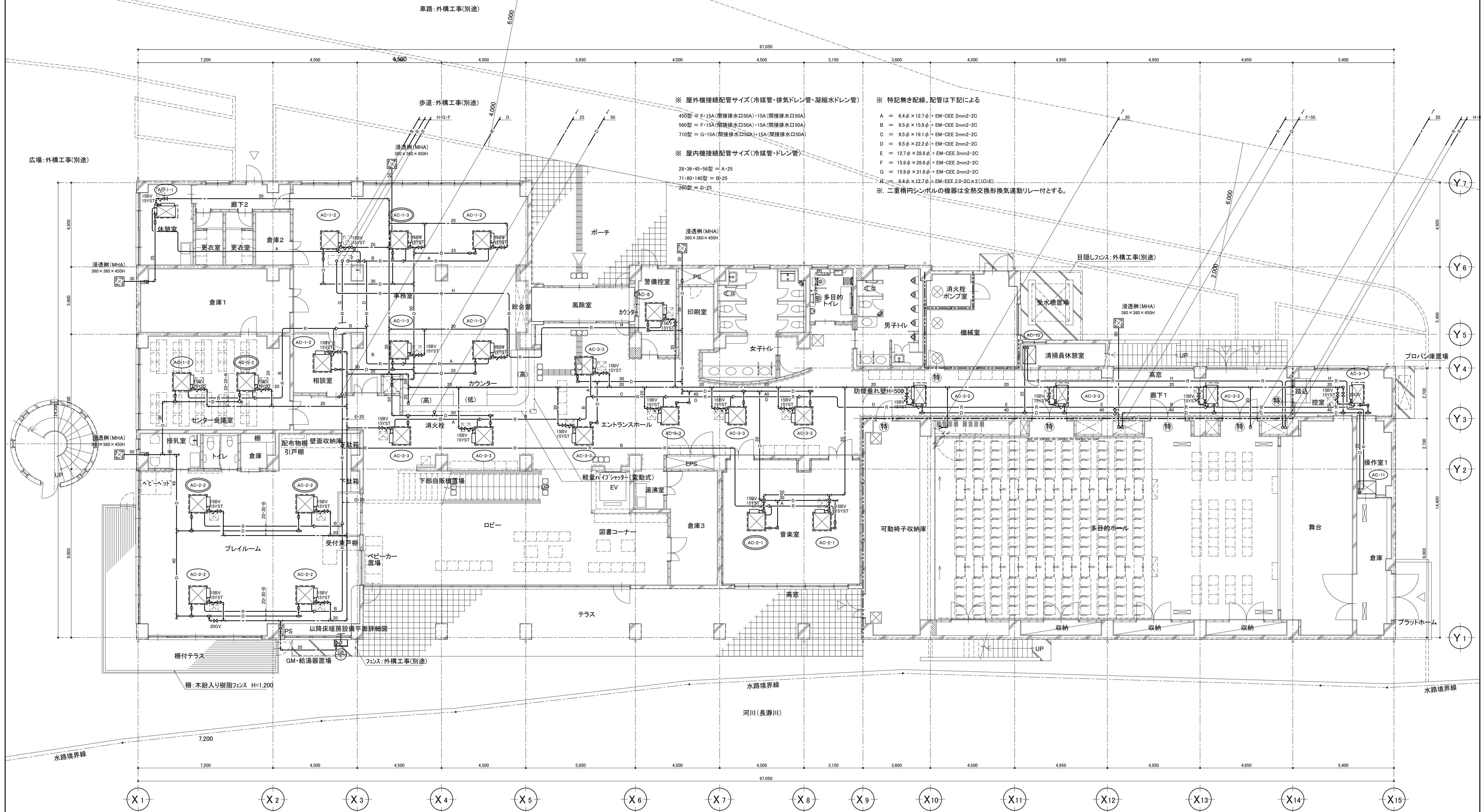
1 階 平 面 図 1:100
