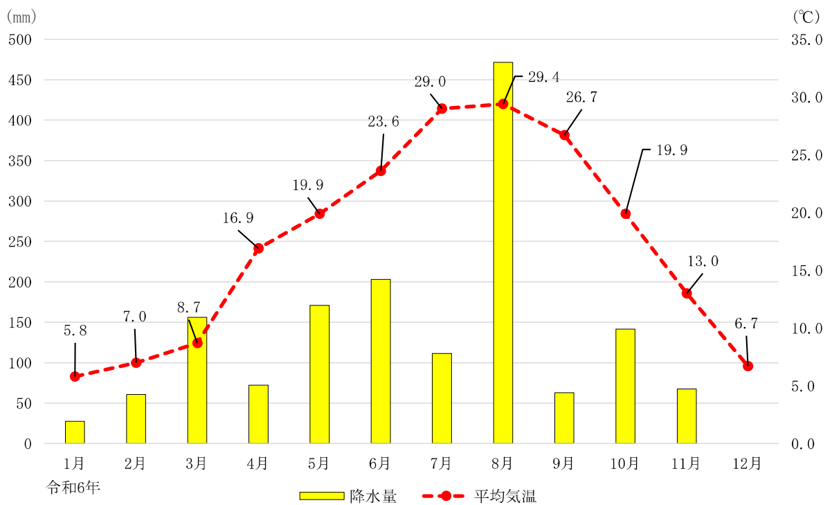
(A-7) 月間降水量と平均気温
