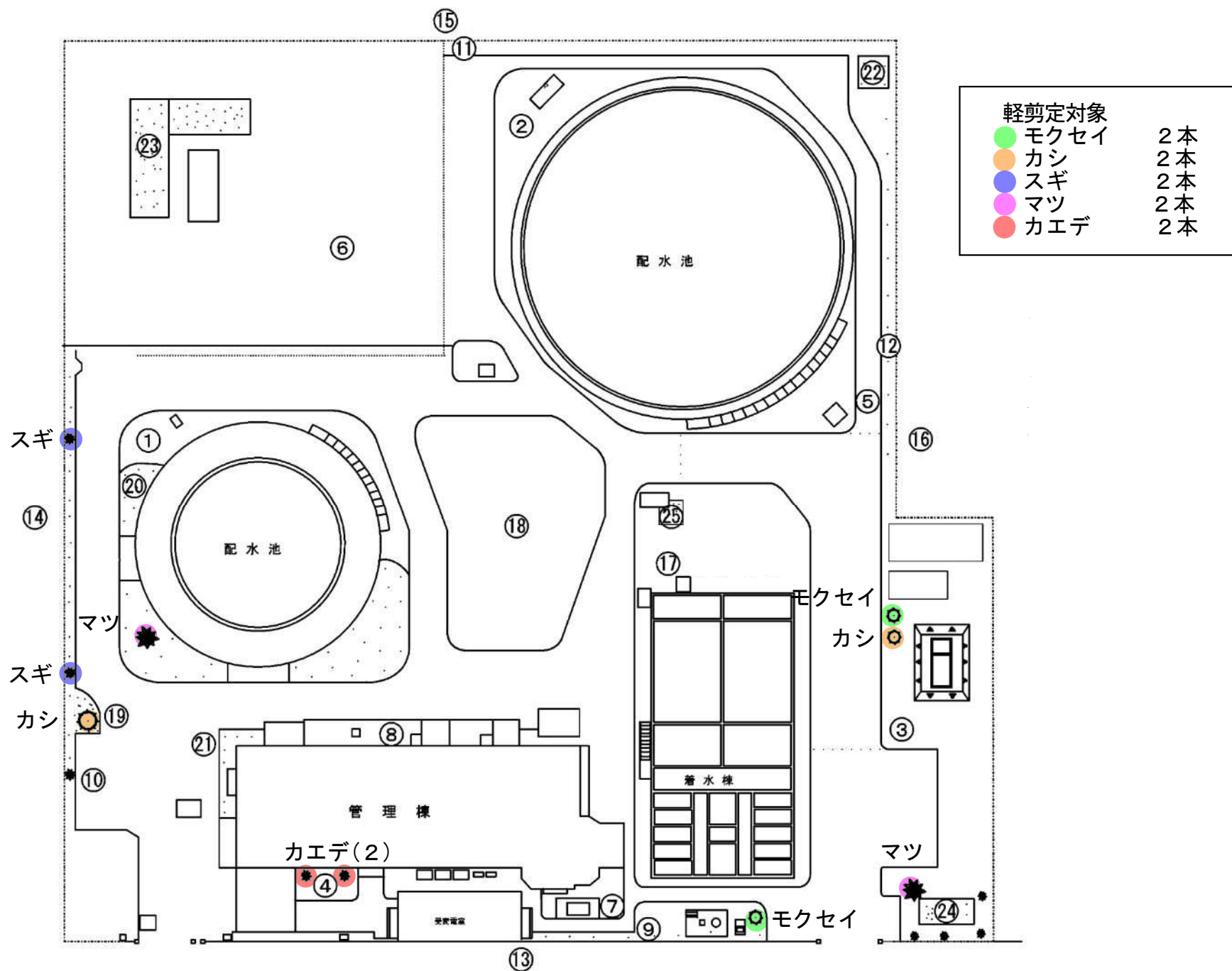
仙波浄水場平面図
