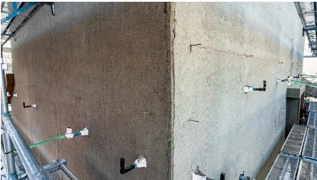
縦縄入れ後の乾燥養生（外壁）
