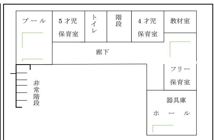
2階平面図
