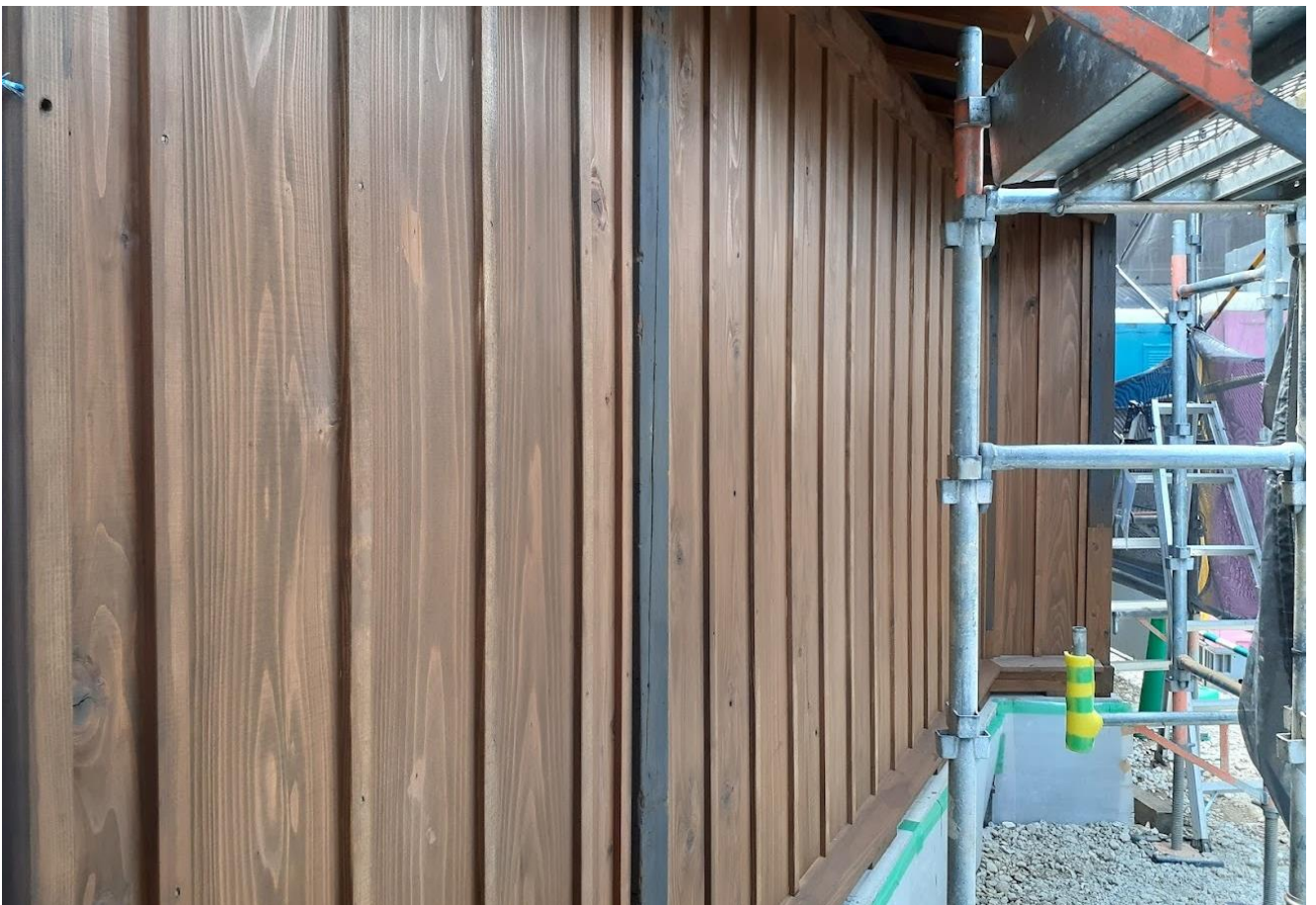
旧栄養食配給所炊事場棟外壁の施工状況
