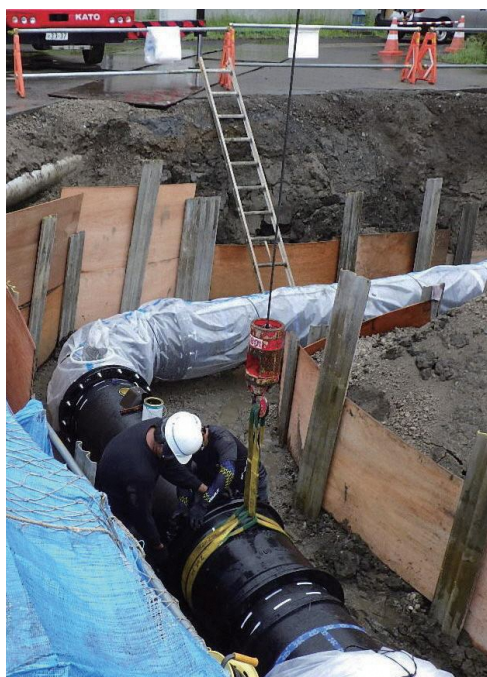
浄水場内の配水管布設工事
