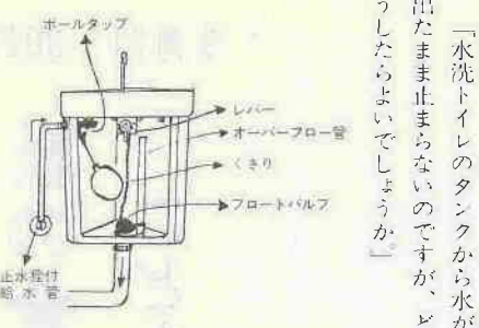
ロータンク内部図
