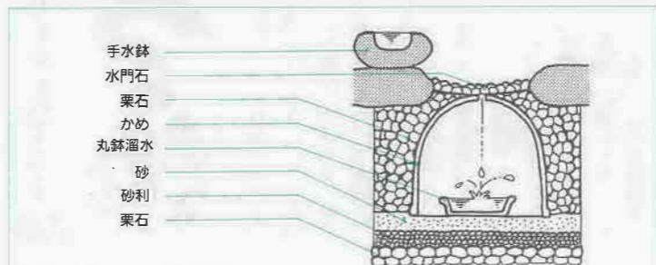
図Ⅱ 水琴窟のしくみ
